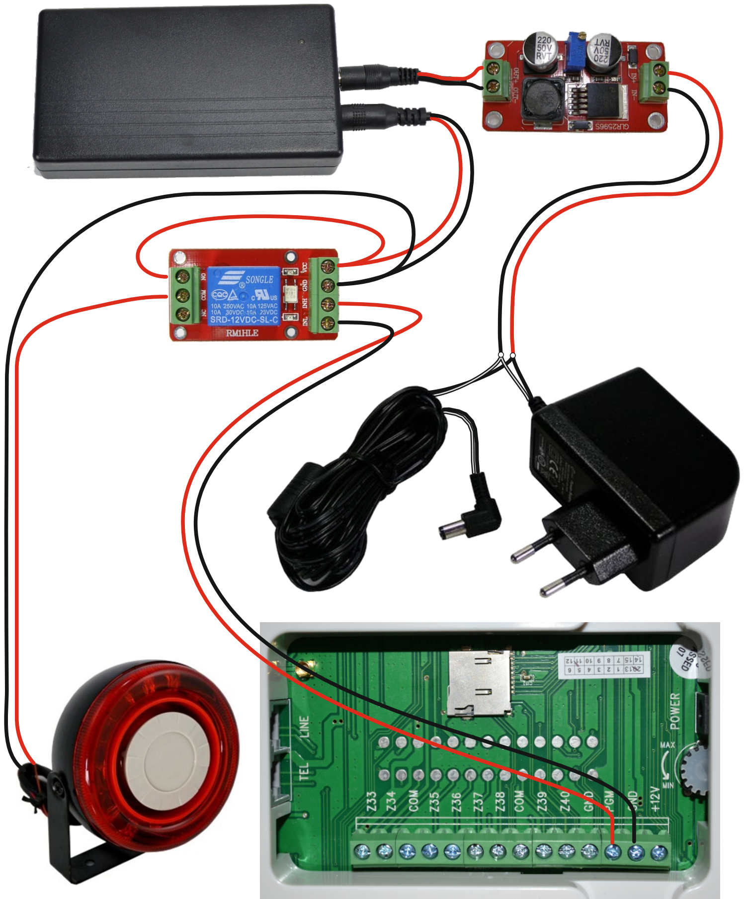
Ekstern sirene til backup forsyning - SSI 500
