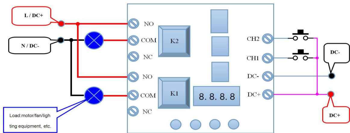
FRM02 参考接线图
