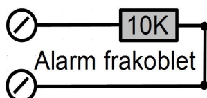
NC Funktion med 10K \Omega
